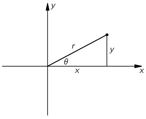
图 22.2: x + iy = re^{i\theta}
