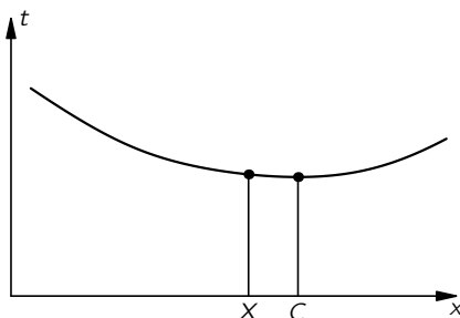
图 26.5: C 点相应于最短时间，但其附近各点相应于几乎与之相同的时间
