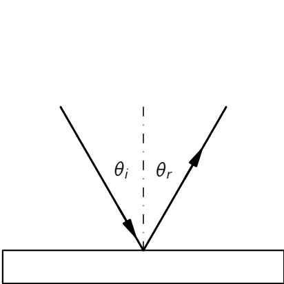
图 26.1: 入射角等于反射角
