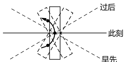
图 20.4: 当图20.2的自旋轮子的轴在转动时，轮子上的质点是沿曲线运动的
