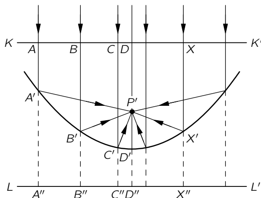
图 26.12: 抛物面镜
