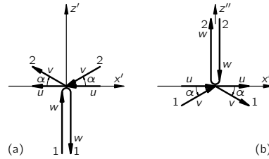
图 16.3: 从运动汽车上看上去的碰撞的另外两种视图
