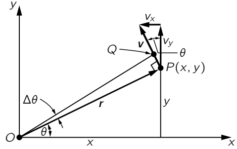
图 18.1: 二维转动动力学图示
