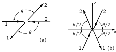
图 16.2: 两个以相等速率、相向运动的相同粒子所发生的弹性碰撞的两种视图
