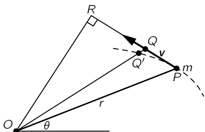
图 18.3: 一个围绕轴 O 运动的质点
