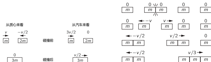
图 10.7: m 和 2m 之间的非弹性碰撞的两种看法 图 10.8: 2m 和 3m 之间的作用与反作用
